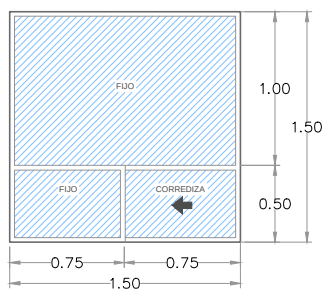
Ventana 1 CRISTAL CLARO DE 4 mm CON MARCO DE ALUMINIO BLANCO VISTA EXTERIOR / ALZADO
