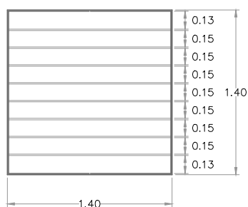
Protección 1 REJA DE PROTECCIÓN EN HERRERIA (COLOR BLANCO) FACHADA PRINCIPAL VISTA EXTERIOR / ALZADO
