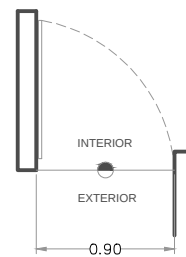
Puerta Principal PROTOTIPO TIPO / FACHADA PRINCIPAL PLANTA
