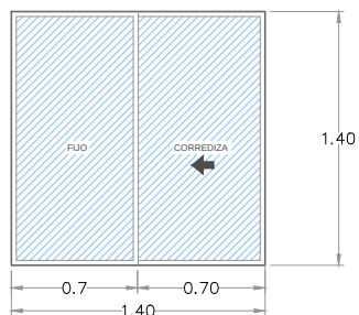
Ventana 1 CRISTAL CLARO DE 4 mm CON MARCO DE ALUMINIO BLANCO VISTA EXTERIOR / ALZADO
