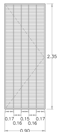
Protección 2 PROTOTIPO TIPO / FACHADA PRINCIPAL VISTA EXTERIOR / ALZADO
